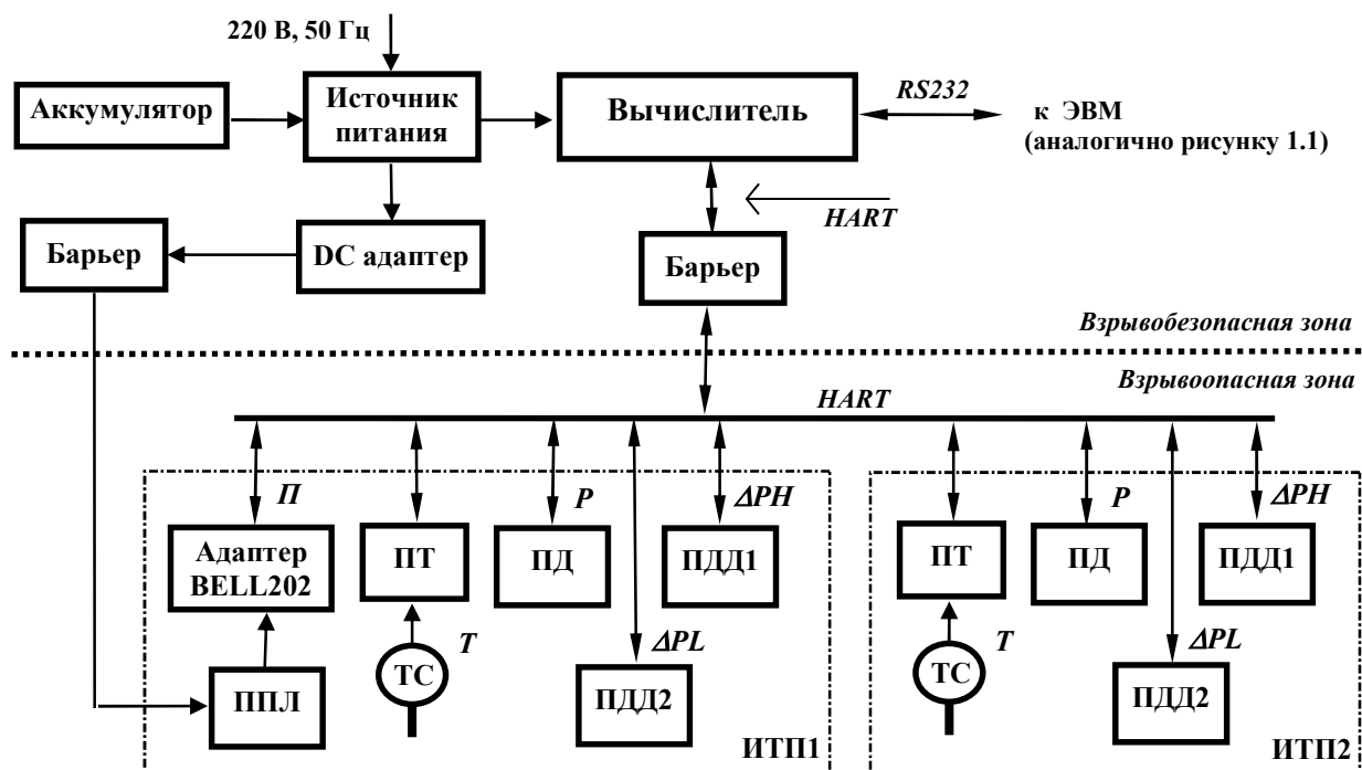
Рисунок 1.7 – Структурная схема Комплексов модификаций ФЛОУТЭК-ТМ-1-1 и ФЛОУТЭК-ТМ-2-1 при обслуживании двух трубопроводов
