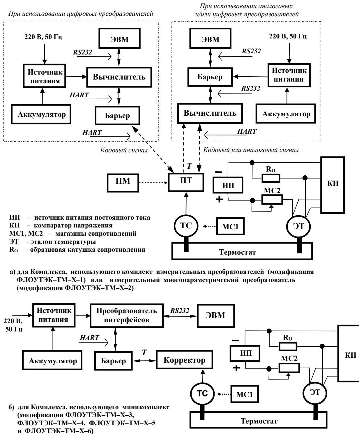
Рисунок 3.10 – Схема для проверки выполнения Комплексами измерений температуры
