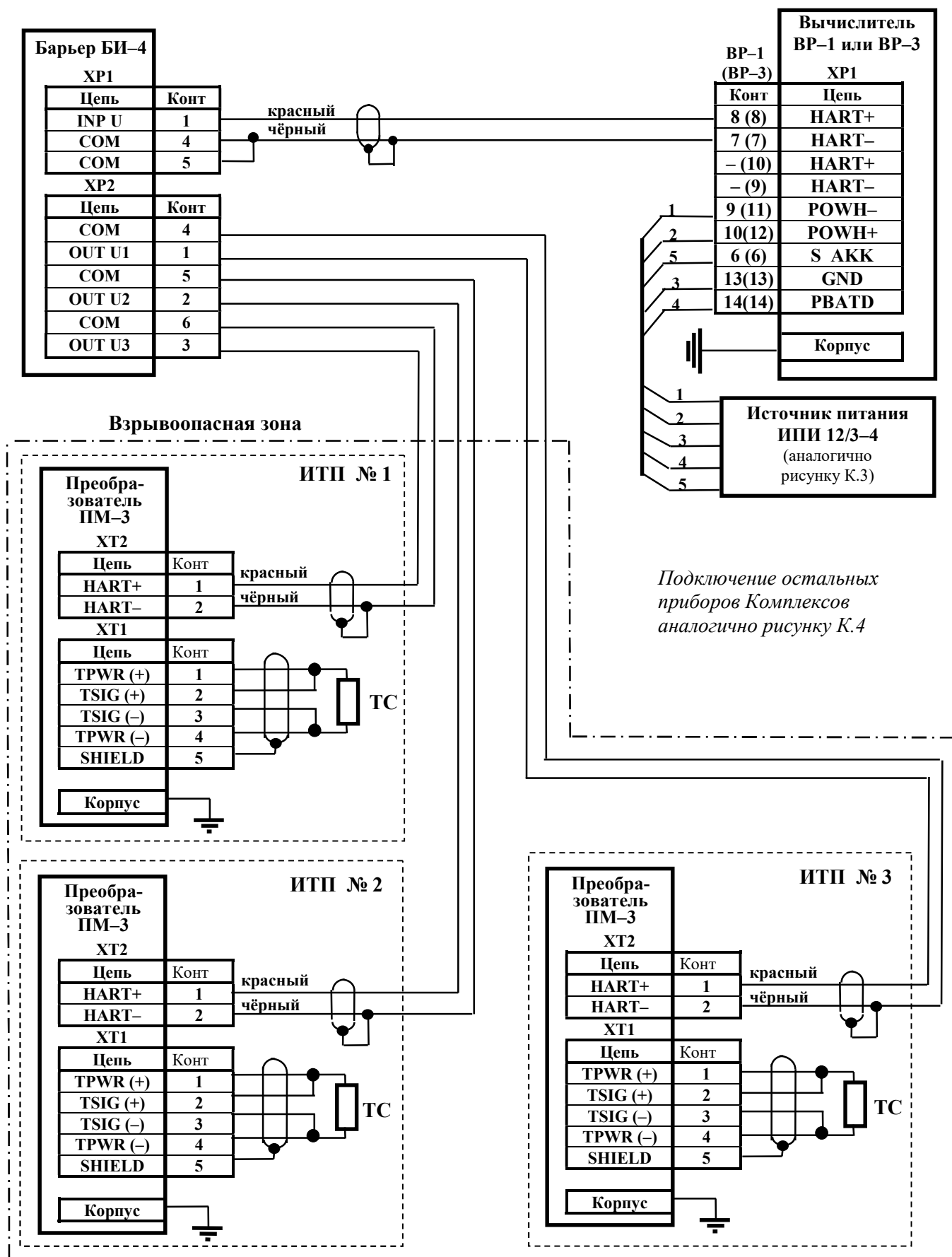
Рисунок К.8 – Схема подключения измерительных многопараметрических преобразователей с кодовыми выходными сигналами к вычислителю Комплексов модификаций ФЛОУТЭК-ТМ-1-2 и ФЛОУТЭК-ТМ-2-2 при обслуживании трех трубопроводов
