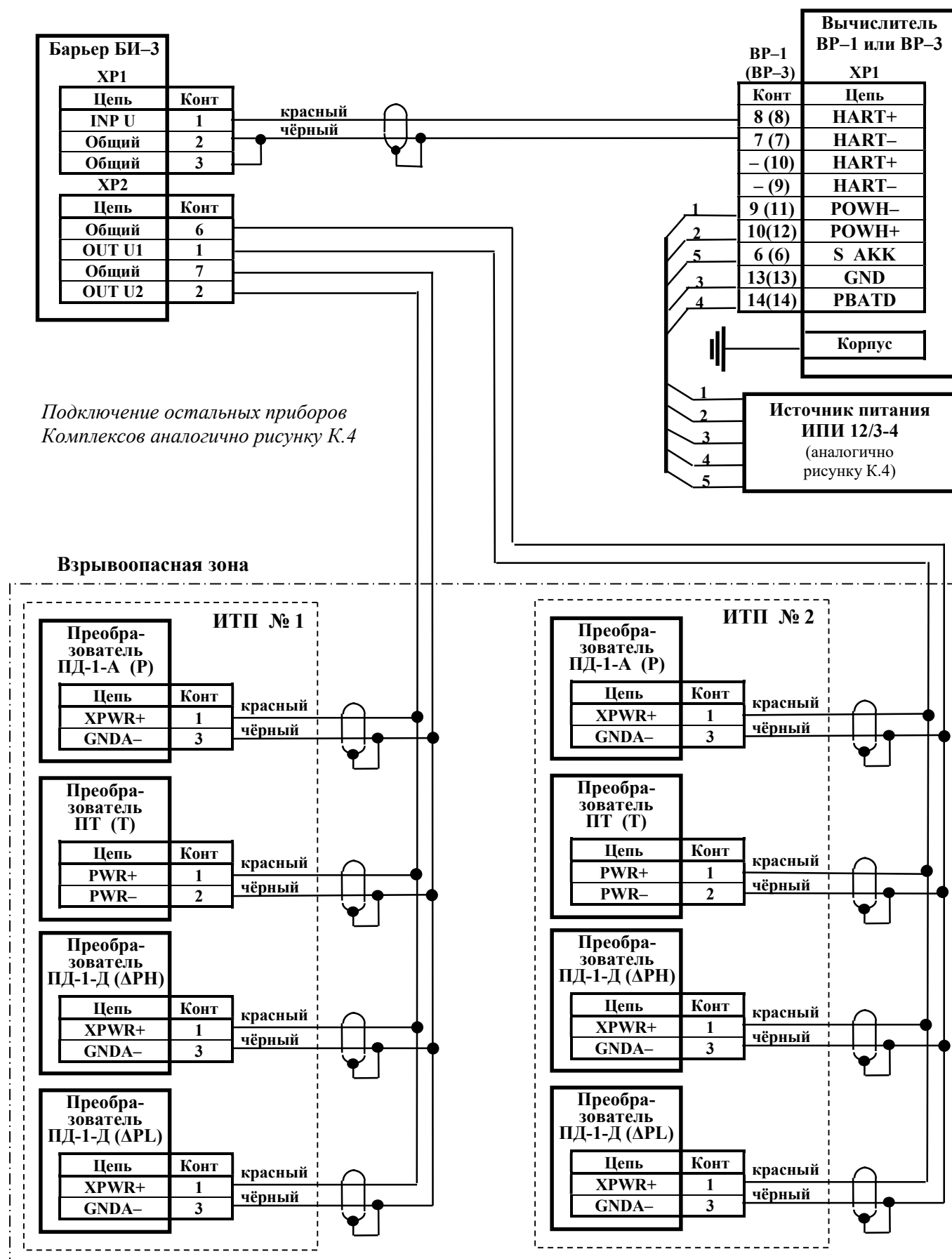
Рисунок К.7 – Схема подключения измерительных преобразователей с кодовыми выходными сигналами к вычислителю Комплексов модификаций ФЛОУТЭК-ТМ-1-1 и ФЛОУТЭК-ТМ-2-1 при обслуживании двух трубопроводов
