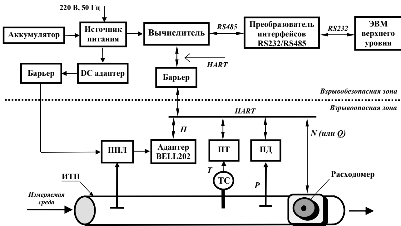
б) Комплекс модификации ФЛОУТЭК-ТМ-4-1 при использовании расходомера с кодовым выходным сигналом
