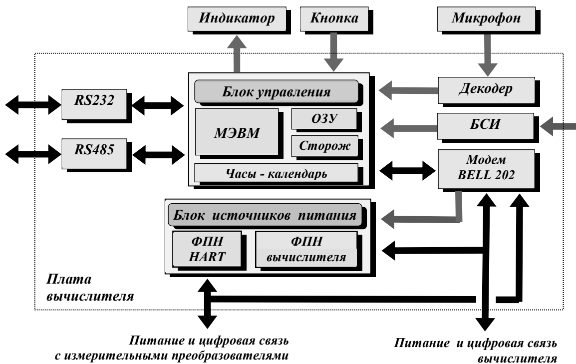
Рисунок 2.2 – Структурная схема вычислителя ВР
