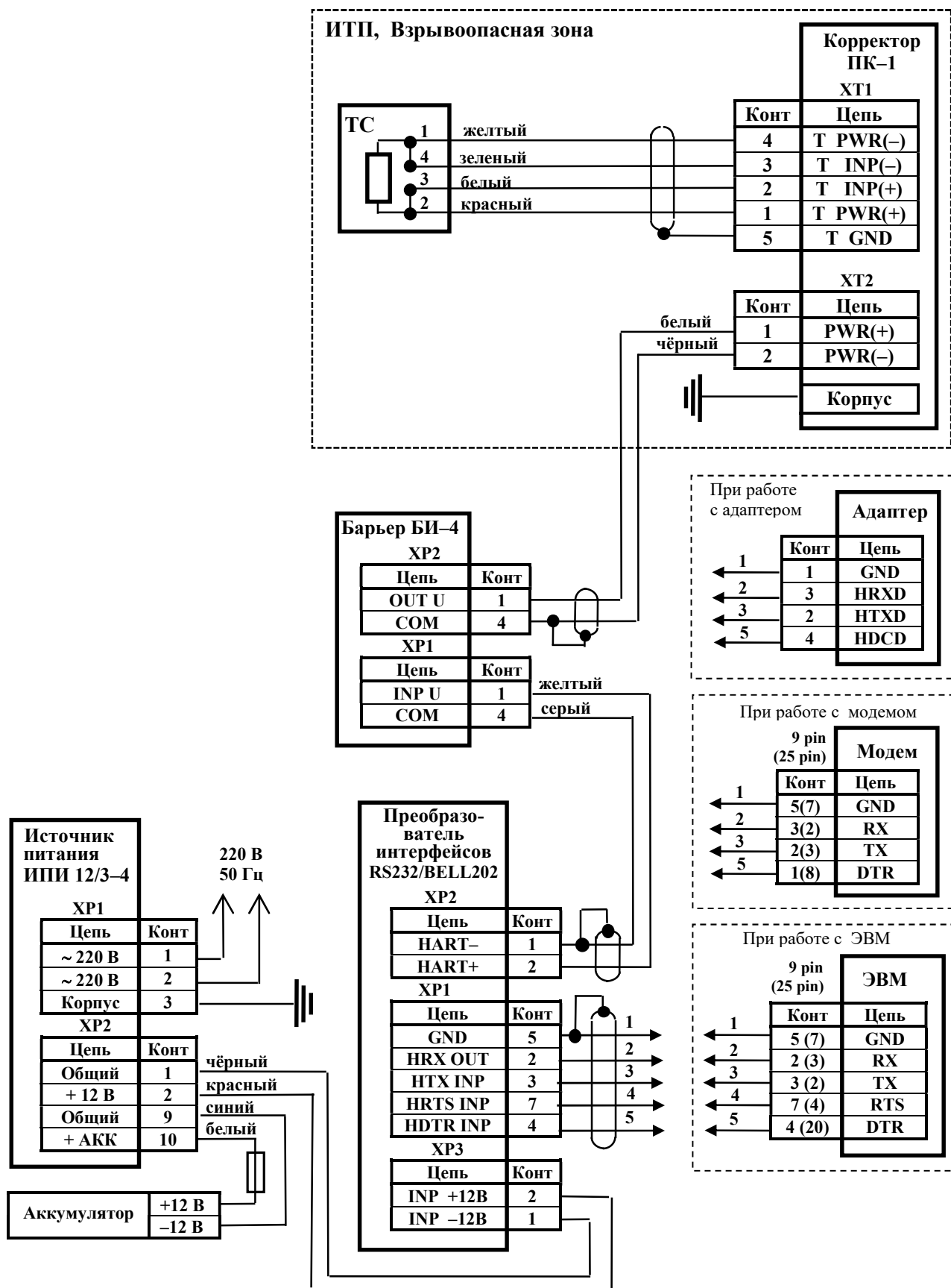
Рисунок К.1 – Схема подключения приборов Комплексов модификаций ФЛОУТЭК-ТМ-1-3 и ФЛОУТЭК-ТМ-2-3 (миникомплексы) при обслуживании одного трубопровода
