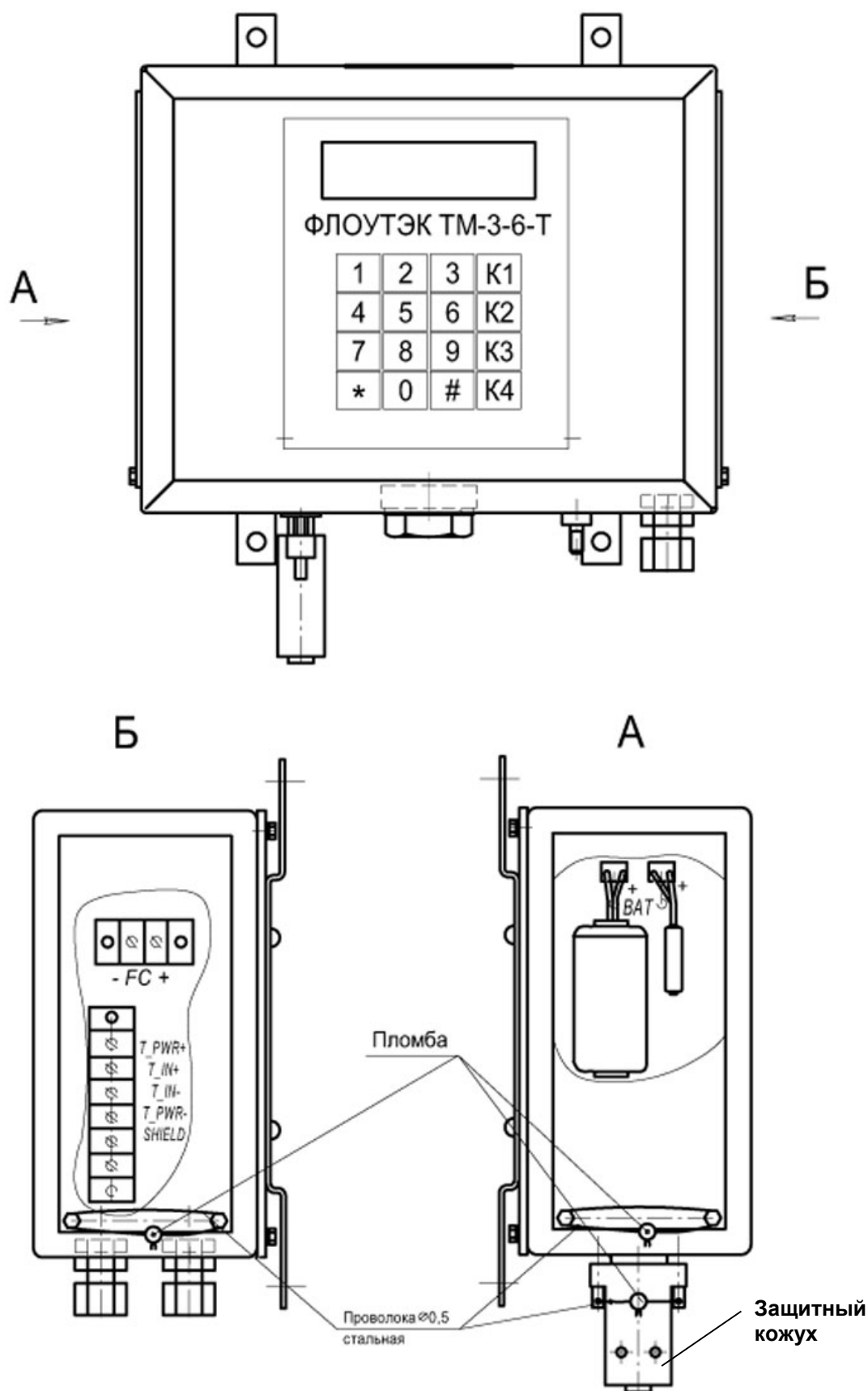
Рисунок Л.4 – Схема размещения пломб на преобразователе – корректоре ПК-3Т (размещение пломб на преобразователе – корректоре ПК-3 аналогично)
