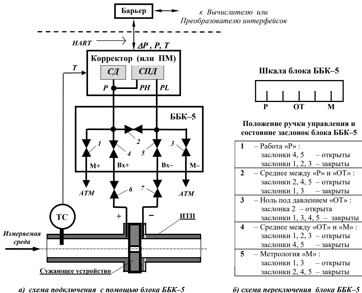
Рисунок 3.7 – Схема подключения корректора (или измерительного многопараметрического преобразователя) Комплексов к одностороннему трубопроводу с помощью блока ББК-5 и схема переключения блока ББК-5
