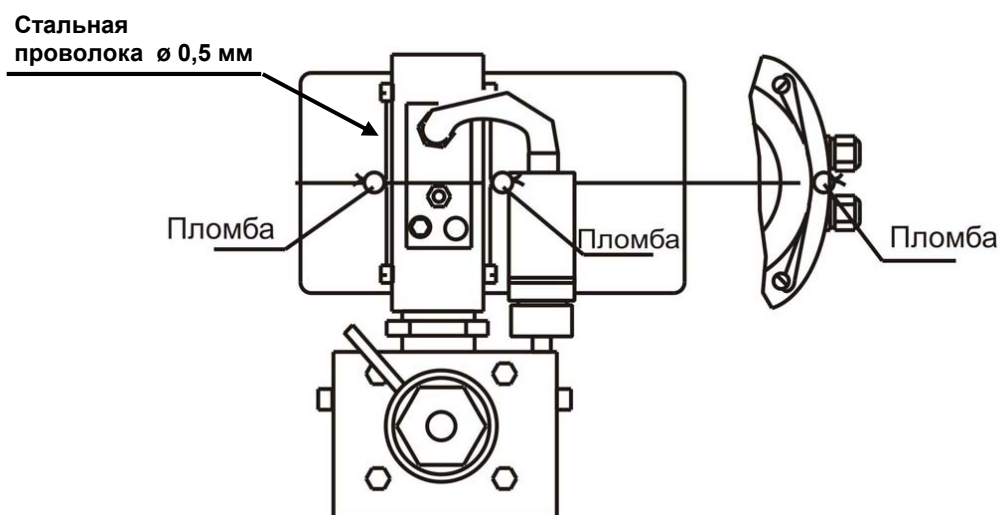
Рисунок Л.2 – Схема размещения пломб на преобразователе – корректоре ПК-1 и на преобразователе давления ПД-1-Д (размещение пломб на преобразователе – корректоре ПК-2 и на преобразователях давления ПД-1-А и ПД-1-И аналогично)
