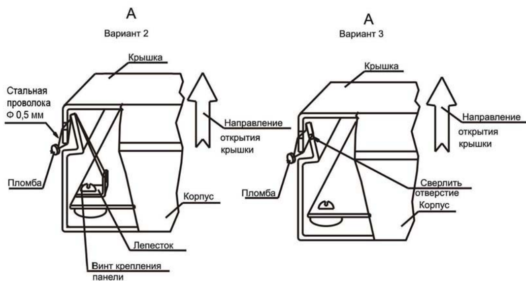
Рисунок Л.3 – Схема размещения пломбы на вычислителе, варианты 1, 2 и 3 (размещение пломб на преобразователе – корректоре ПК-4 аналогично)
