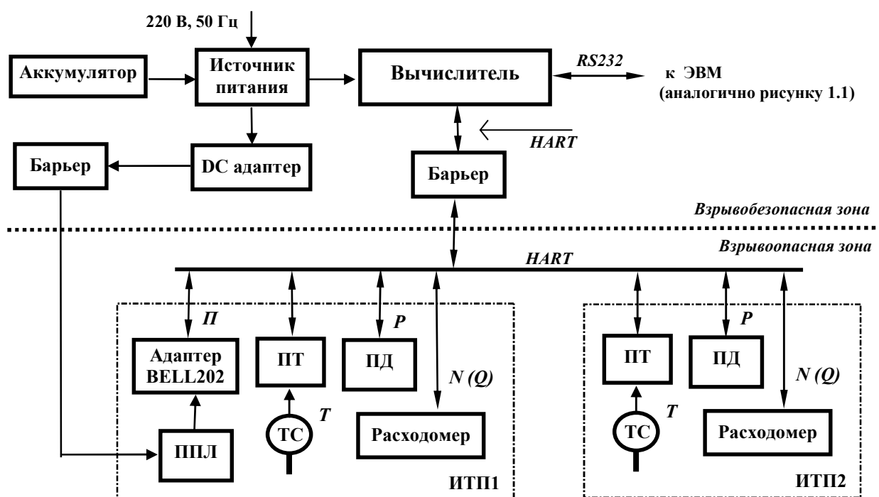
Рисунок 1.8 – Структурная схема Комплексов модификации ФЛОУТЭК-ТМ-4-1 при обслуживании двух трубопроводов и использовании расходомеров с кодовым выходным сигналом
