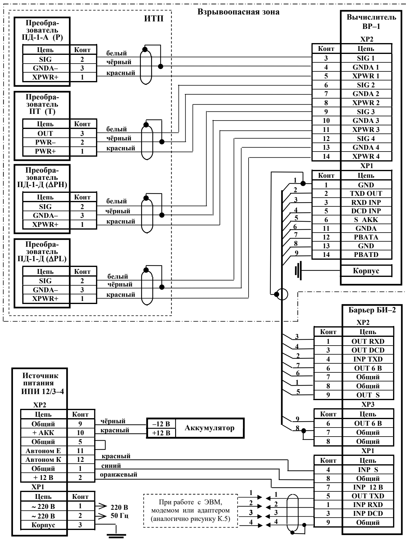
Рисунок К.6 – Схема подключения вычислителя Комплексов модификаций ФЛОУТЭК-ТМ-1-1 и ФЛОУТЭК-ТМ-2-1 при обработке аналоговых сигналов и при обслуживании одного трубопровода
