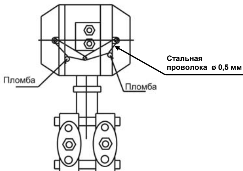
Рисунок Л.1 – Схема размещения пломбы на многопараметрическом преобразователе – вычислителе ПМ-3
